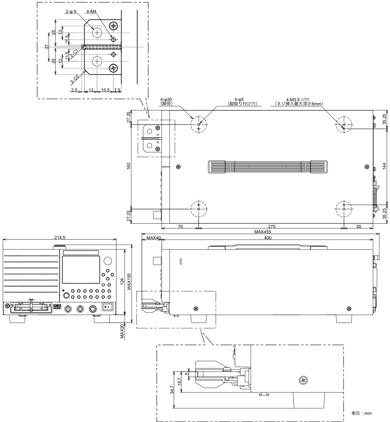
外形図 (PLZ164WL, PLZ334WL)
